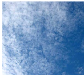
Cirrocumulus
